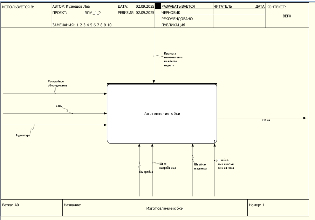
Рисунок 3 – Диаграмма процесса изготовления юбки
